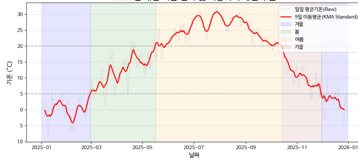
2025년 대전 기온 변화 및 기상학적 계절 구분
