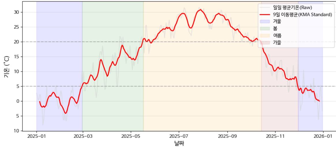
2025년 거제 기온 변화 및 기상학적 계절 구분
