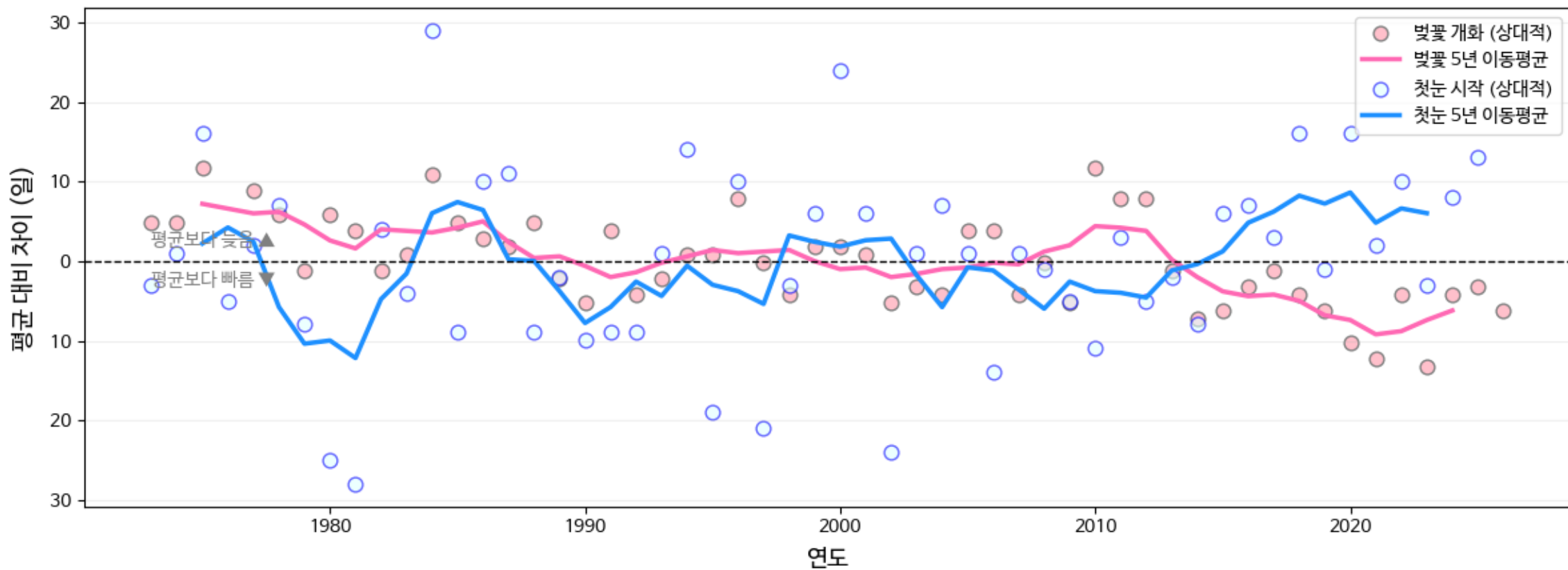
충남대학교 벚꽃 개화 및 첫눈 시기 변화
