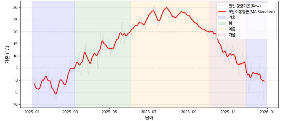
2025년 거제 기온 변화 및 기상학적 계절 구분
